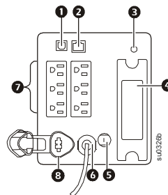
500/750 ВА 100 В переменного тока 750 ВА 120 В переменного тока
