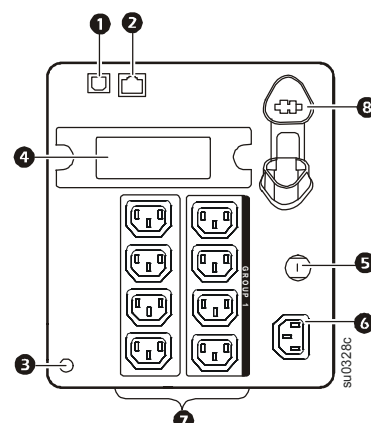
1000/1500 ВА 230 В переменного тока
